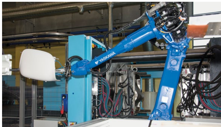
Billederne viser SP Mouldings nye 1.300 tons maskine i arbejde på fabrikken i Juelsminde
